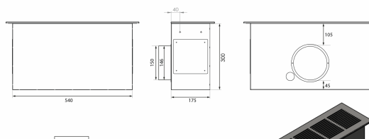
Plasmex®-filter skjuler, Indbygning over skab - Hybrid - Rev. 2
